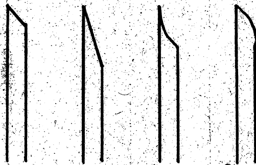
zu stumpfer Winkel zu spitzer Winkel Hohl geschliffen Rund geschliffen
