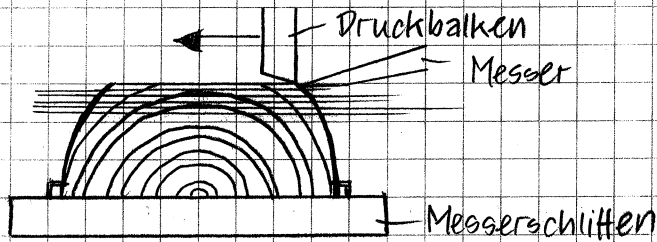
Flachmessern horizontal
