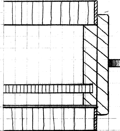
4) überfälzt
