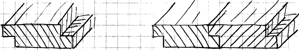
überfälzte Fuge
