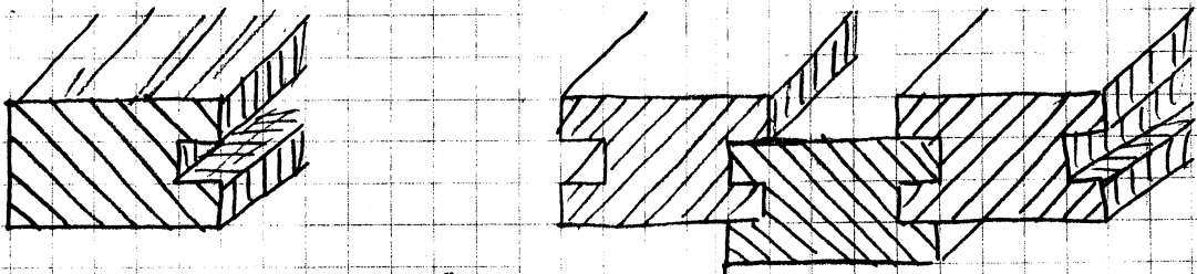
überschiebende Schalung
