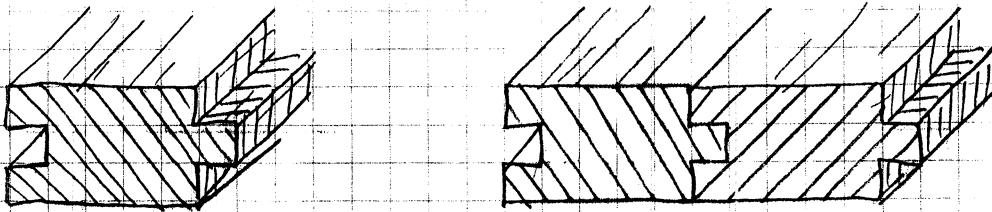
gespundete Fuge
